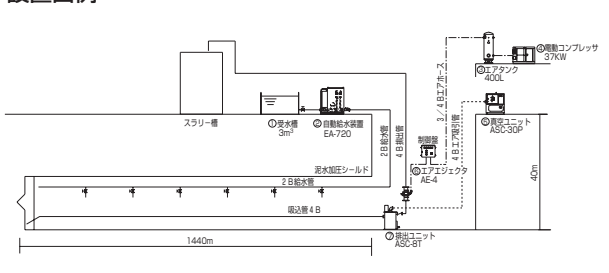
設置図例
