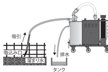
ミニバキューマー使用例 コンクリート打設現場
